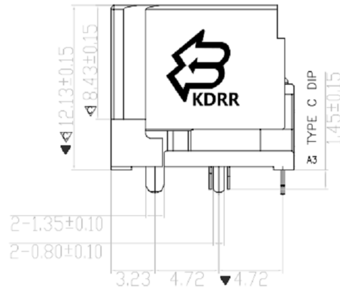
截面 A-A
