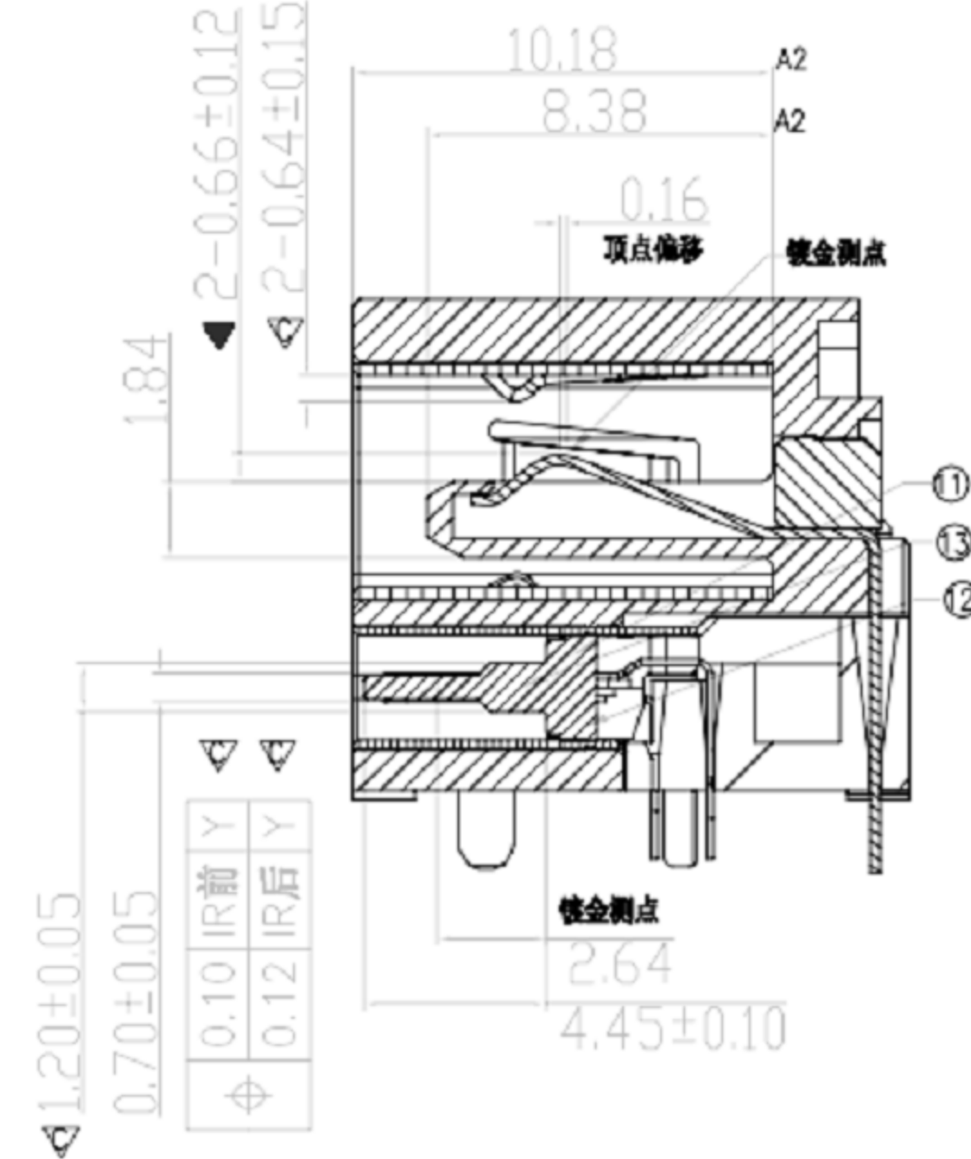
截面 A-A
